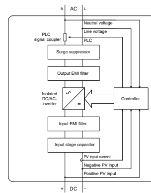
IQ9N Microinverter
