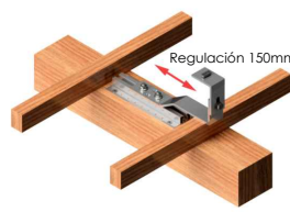
Anclaje atornillado
